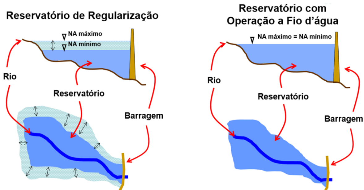
Figura 4 – Tipo de Reservatório
