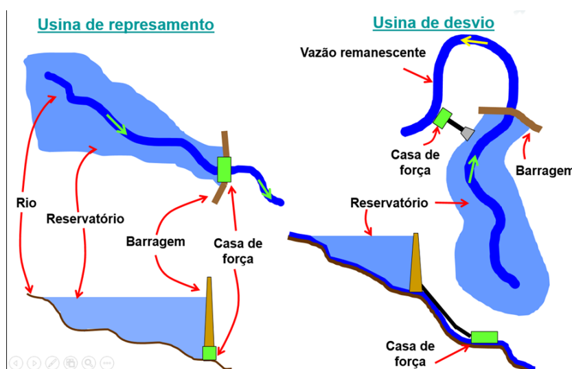
Figura 3 – Tipo de Arranjo
