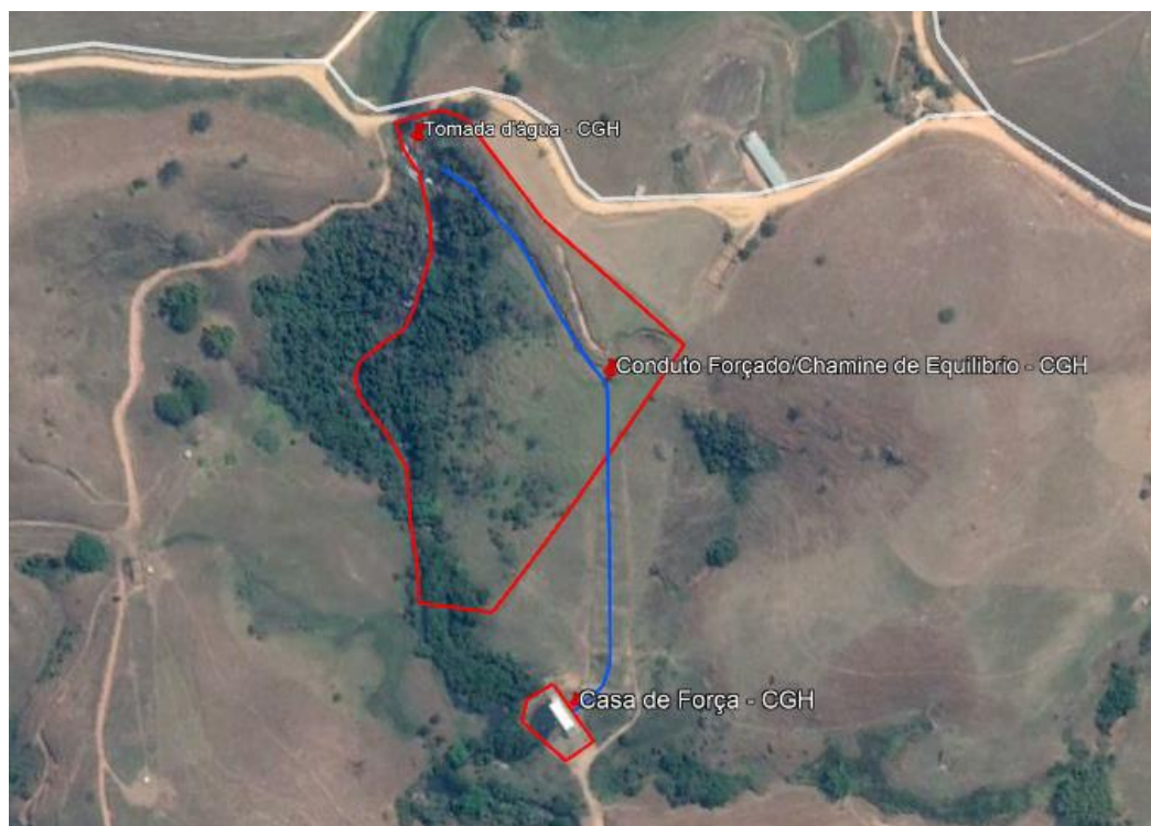
Figura 6 – Arranjo de um CGH
