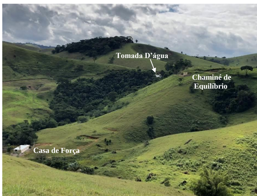
Figura 7 – Foto do arranjo de uma CGH
